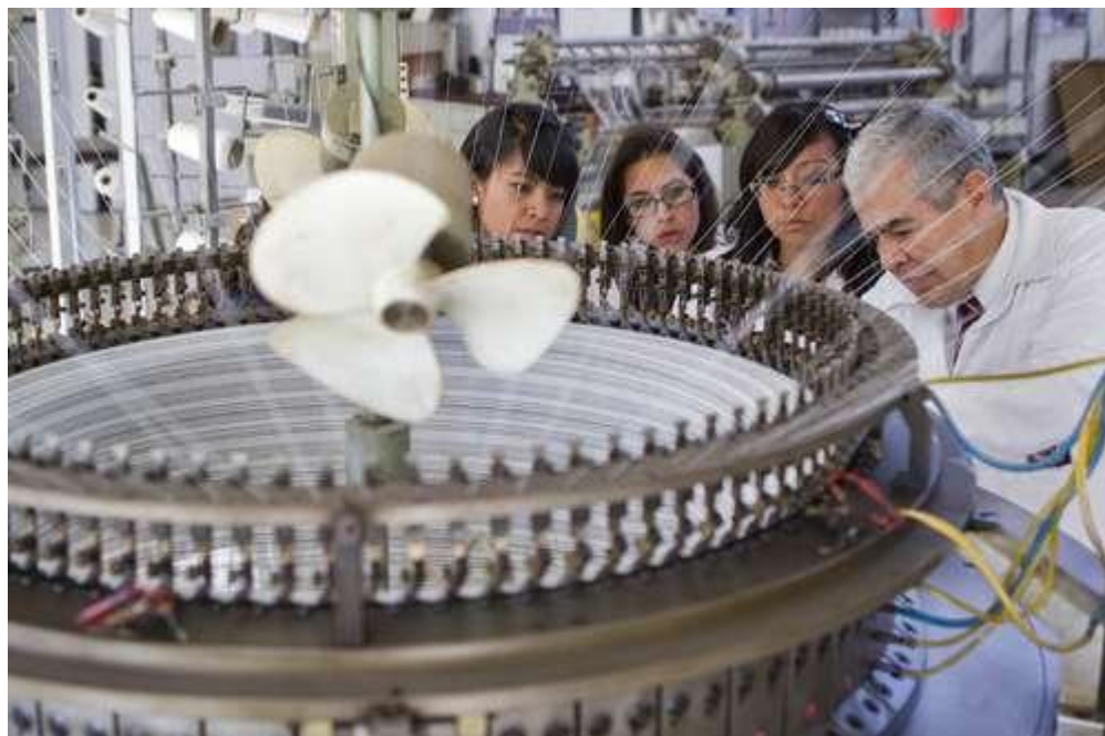
Laboratorio de tejido de punto de la Escuela Superior de Ingeniería Textil. Foto José Carlo González
